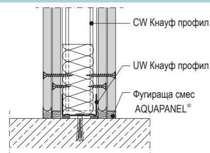
W382.bg-VU1 Връзка към под
