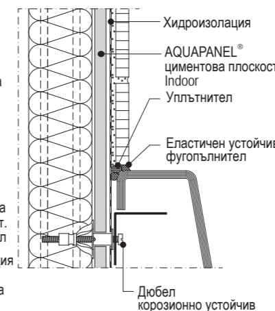
W381.bg-ZH4 Контакт на стена и вана
