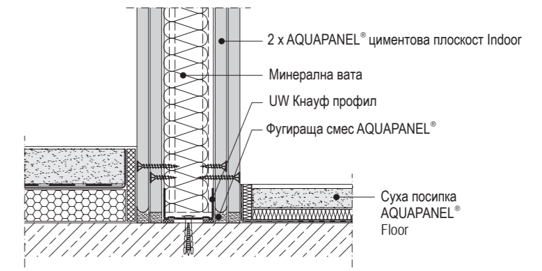
W386.bg-VU3 Връзка към плоча
