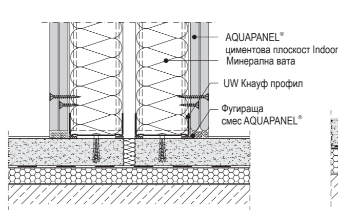
W381.bg-V03 Плаваща връзка
