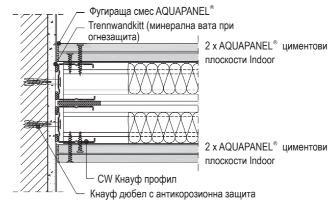
Детайли М 1:5
