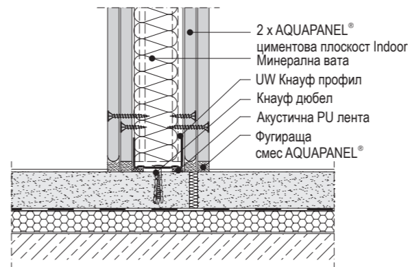
W386.bg-VU2 Закрепване върху финалната настилка
