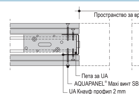
W382.bg-E1 Врата окантена с UA профил
