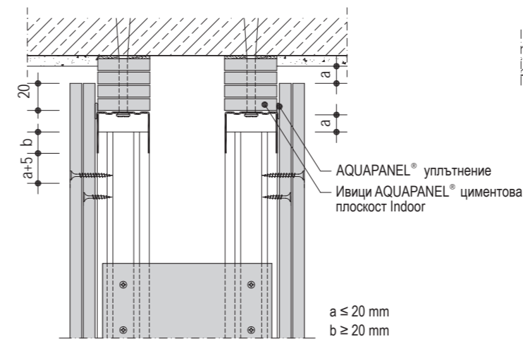
W382.bg-ZH1 Тръбно преминаване
