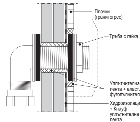
W382.bg-ZH1 Тръбно преминаване
