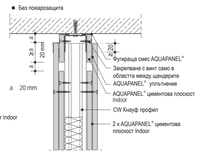
W385.bg-V02 Плъзгаща връзка към таван
