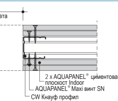
W382.bg-E1 Врата окантена с CW профил
